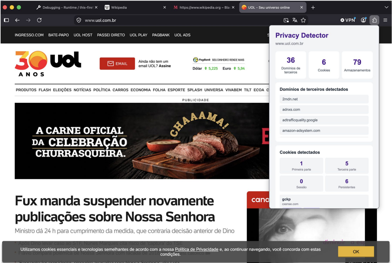
Figura 22 - UOL: resumo e domínios de terceiros.
